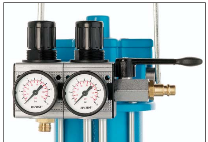
Сдвоенный регулятор сжатого воздуха для создания давления распыления и регулирующего воздушного потока у воздушно-комбинированных версий
